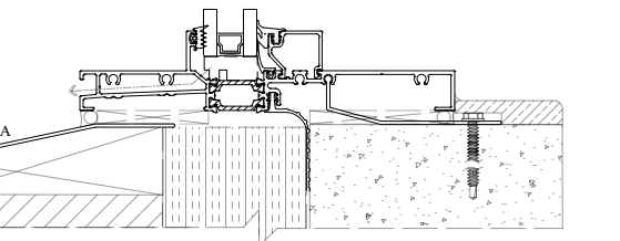
3B OPTIONAL SILL w/ EXTENDED SILL & TREMCO PROGLAZE ETA
