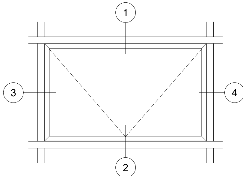
ÉLÉVATION TYPIQUE 4-BAR / VERROUILLAGE MULTIPPOINTS MOUSTIQUAIREEN OPTION
