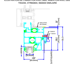
5B TÊTE INSERTION MUR-RIDEAU
