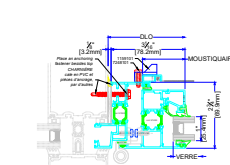
7B JAMBAGE-CÔTÉ CHARNIÈRE INSERTION MUR-RIDEAU
