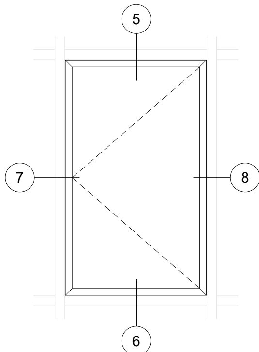
ÉLÉVATION TYPIQUE CHARNIÈRE / ROTO-VERROUILLAGE MULTIPOINTS MOUSTIQUAIRE EN OPTION
