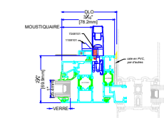
8B JAMBAGE-CÔTÉ VERROU INSERTION MUR-RIDEAU
