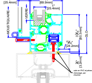
2A SEUIL INSERTION FAÇADE DE MAGASIN
