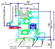
2 SEUIL INSERTION PATTES ÉGALES
