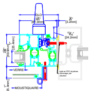
4A JAMBAGE INSERTION FAÇADE DE MAGASIN
