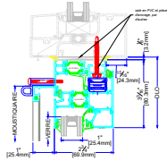
1A TÊTE INSERTION FAÇADE DE MAGASIN
