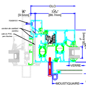
3 JAMBAGE INSERTION PATTES ÉGALES
