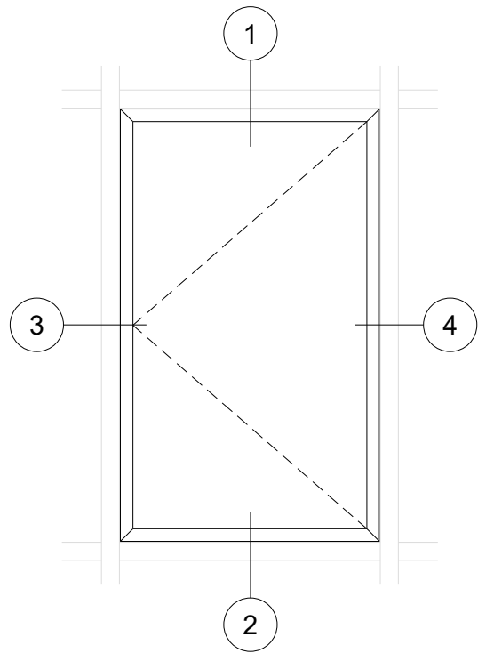
ÉLÉVATION TYPIQUE 4-BAR/ VERROUILLAGE MULTIPOINTS MOUSTIQUAIRE EN OPTION
