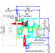
3A JAMBAGE INSERTION FAÇADE DE MAGASIN
