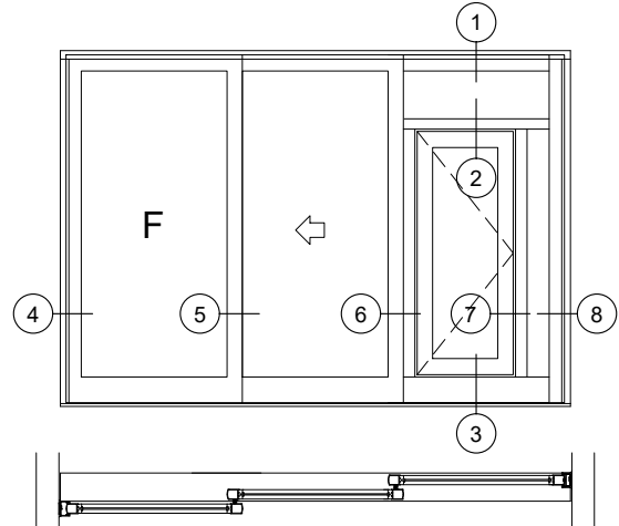
TYPE 'D' ( "MAN" DOOR) / PORTE DE SORTIE
