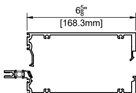
Capped double glazed Couvercles à enclenchement double vitrage
