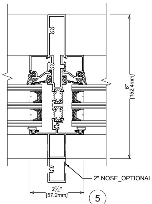
MULLION / MENEAU
