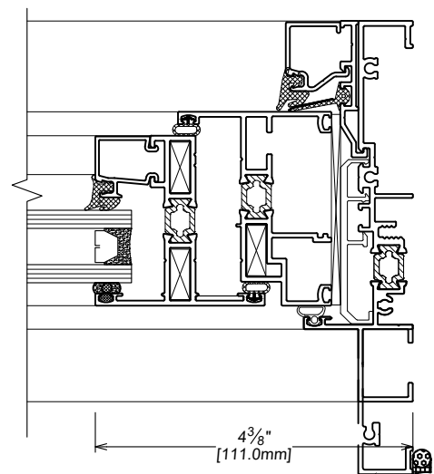
JAMB / JAMBAGE
