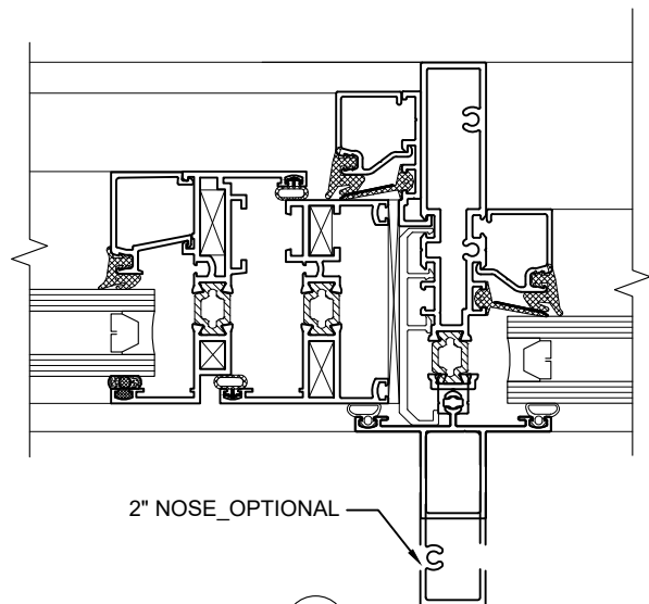
10 MULLION / MENEAU
