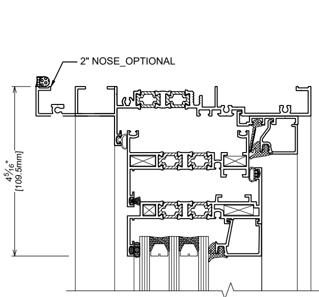
7 HEAD / TÊTE
