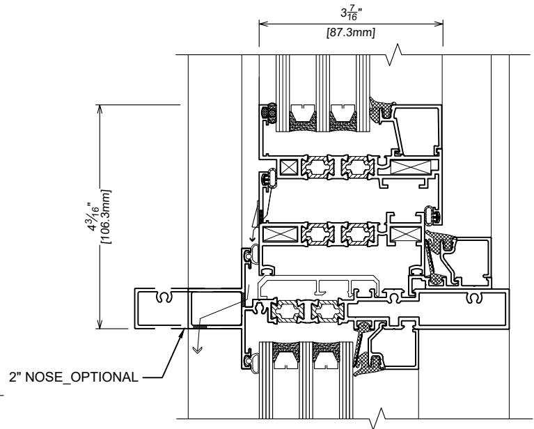
8 HORIZONTAL TRAVERSE HORIZONTALE
