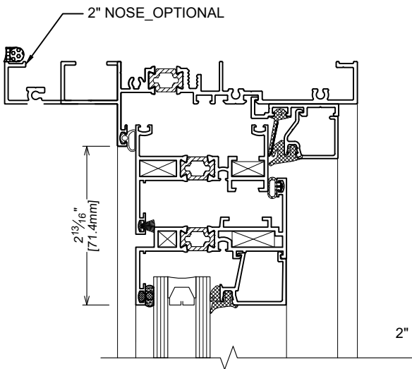
7 HEAD / TÊTE
