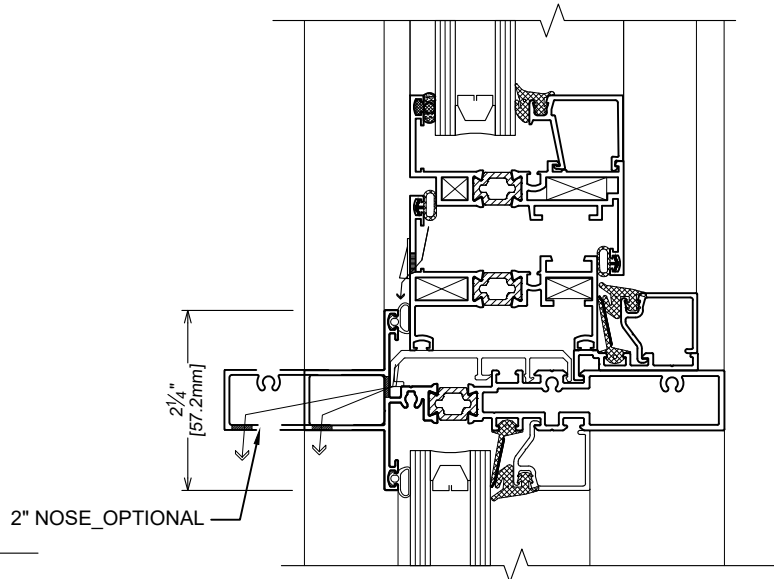
8 HORIZONTAL TRAVERSE HORIZONTALE
