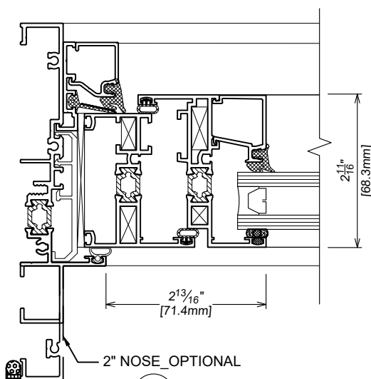
9 JAMB / JAMBAGE
