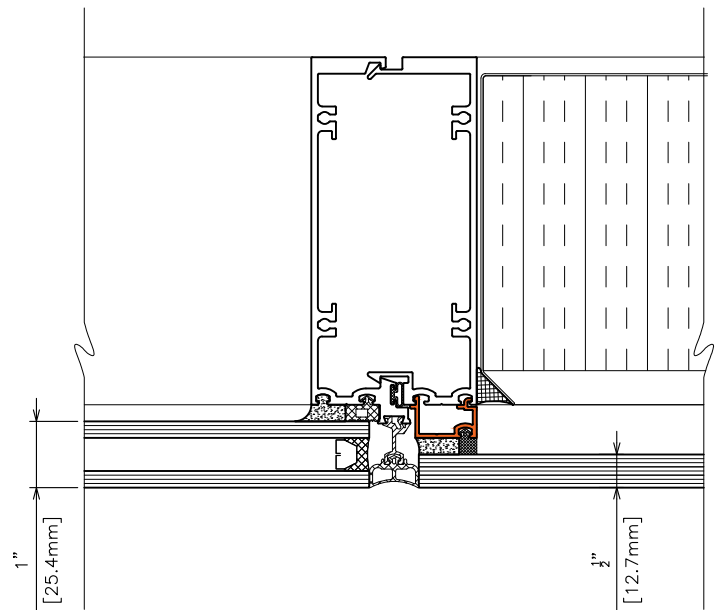
SSG SYSTEM - DOUBLE GLAZED SYSTÈME VSS - DOUBLE VITRAGE
