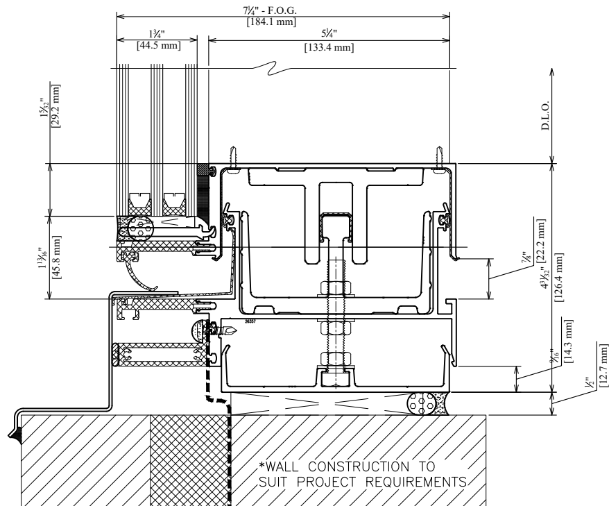
22b HORIZONTAL TRAVERSE HORIZONTALE
