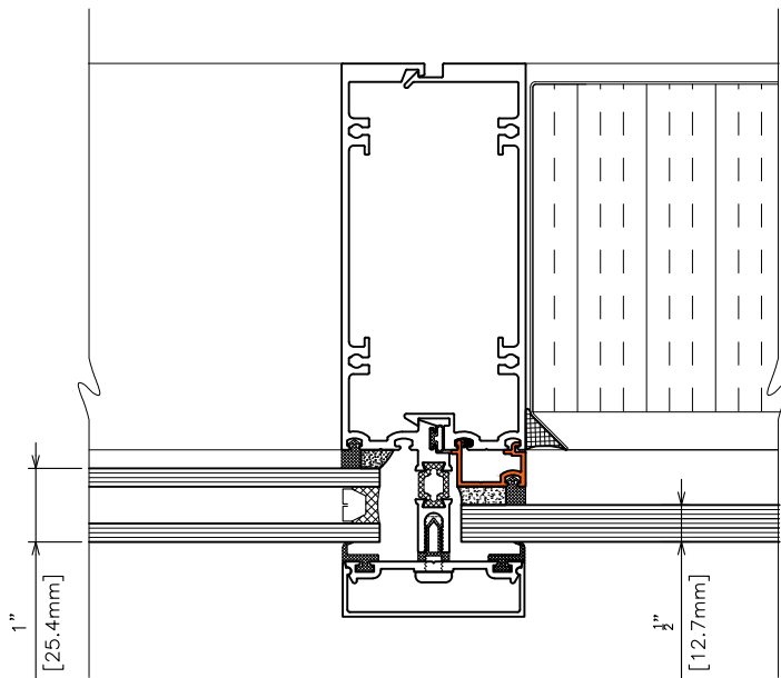
CAPPED SYSTEM SYSTÈME COUVERCLES À ENCLÈCHEMENT
