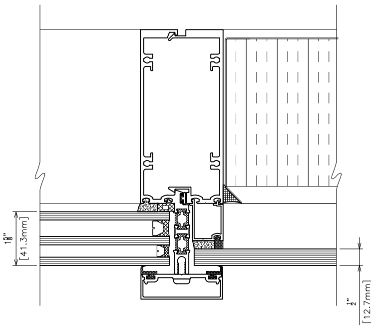
CAPPED SYSTEM SYSTÈME COUVERCLES À ENCLÈCHEMENT
